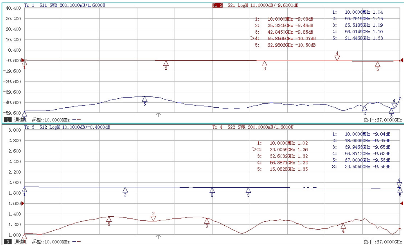
典型曲线
